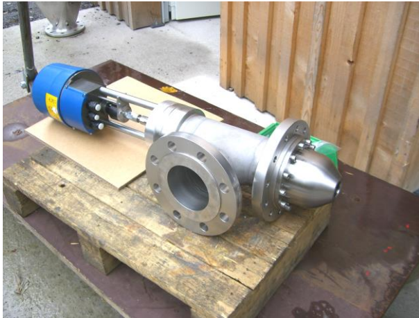
Bypassdüse
